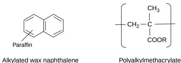
FIGURE 19.32 Examples of pour point depressants.
