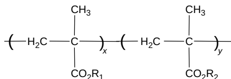
FIGURE 11.8 PMA pour point depressant.
