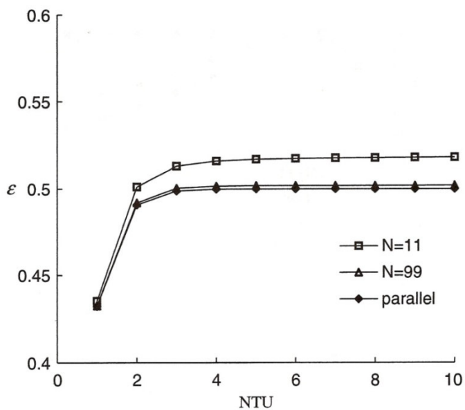
شکل ۹-۱۲: رابطه \epsilon و NTU در چیدمان شماره ۲۲۳ در R=1
