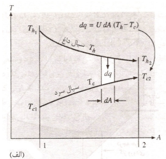
شکل ۱-۱۲: تغییرات دما در طول مبدل برای جریان همسو
