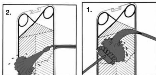
شکل ۹-۴-۱- شستشو با برس نرم و آب روان ۲- شستشو با آب تحت فشار
