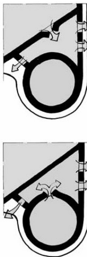
شکل ۱-۳: نحوه قرار گرفتن گسکت‌ها
