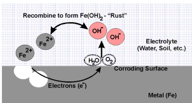
شکل ۸-۹- مکانیسم خوردگی آهن
