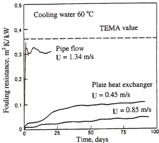
شکل ۵-۹) مقایسه میزان رسوب گرفتگی بین مبدل‌های صفحه‌ای و پوسته و لوله
