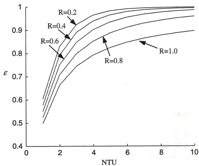
شکل ۱۱-۱۲: رابطه \varepsilon و NTU در چیدمان شماره ۲۲۱ برای تعداد زیاد صفحات
