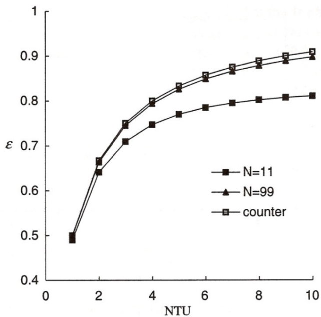
شکل ۱۰-۱۲: رابطه \varepsilon و NTU در چیدمان شماره ۲۲۱ در R=1
