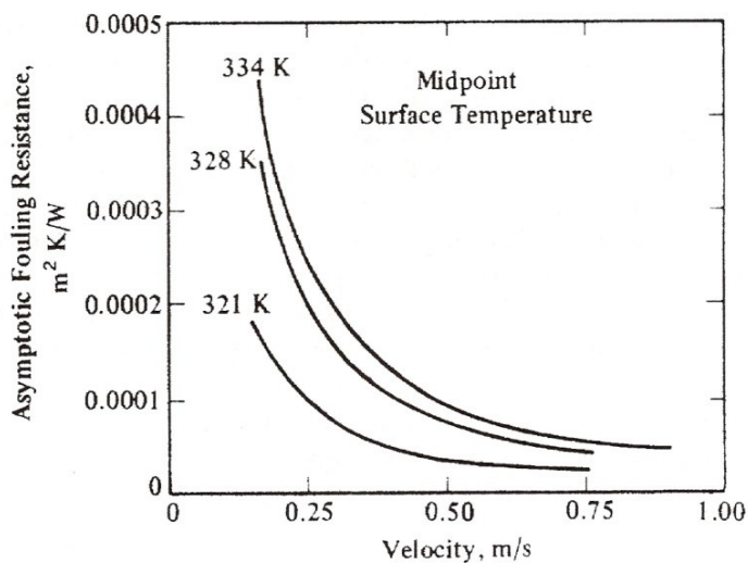
شکل ۵-۹) تاثیر سرعت و دما بر مقاومت انتقال حرارت
