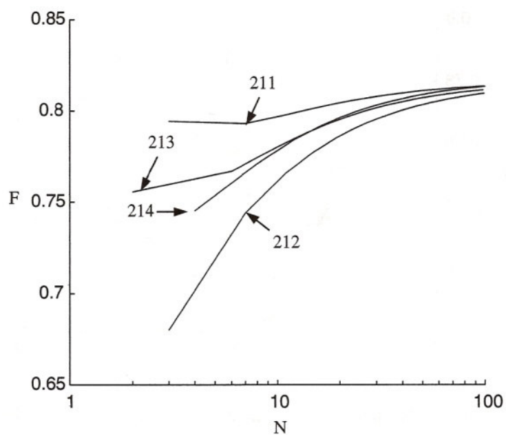
شکل ۴-۱۲: ضریب تصحیح برای چیدمان ۲-۱ در R=0.5 و NTU=2
