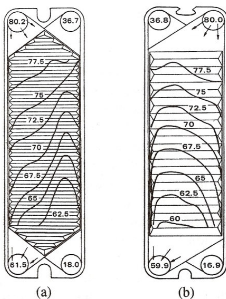
شکل ۷-۲: توزیع جریان و دما در کانالها
