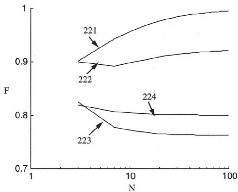
شکل ۵-۱۲: ضریب تصحیح برای چیدمان ۲-۲ در R=0.5 و NTU=1
