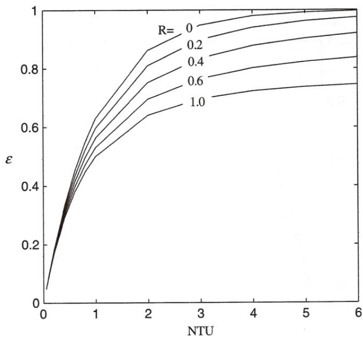
شکل ۱۲-۱۳: رابطه \epsilon و NTU در چیدمان شماره ۳۱۱ برای تعداد زیاد صفحات
