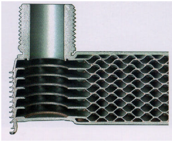
شکل ۵-۲: مبدل صفحه‌ای Brazed
