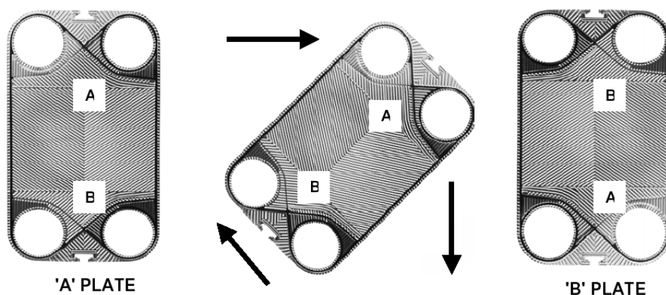
شکل ۵-۶ چگونگی قرارگیری صفحات نسبت به هم
