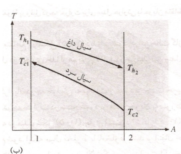
شکل ۱-۱۲: تغییرات دما در طول مبدل برای جریان ناهمسو
