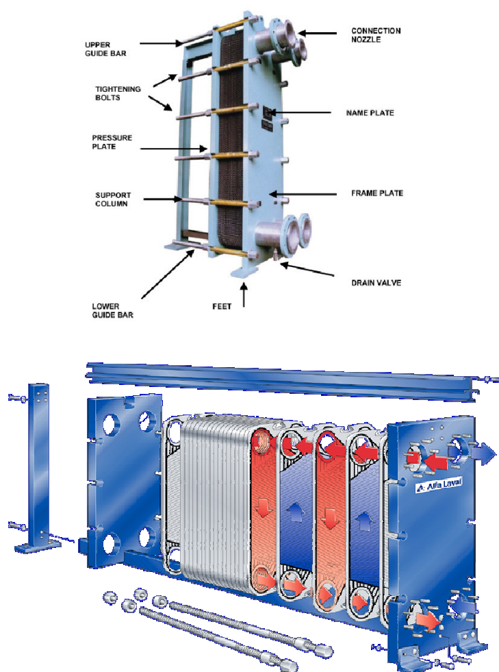
شکل ۲-۱) شمایی کلی از یک مبدل صفحه ای
